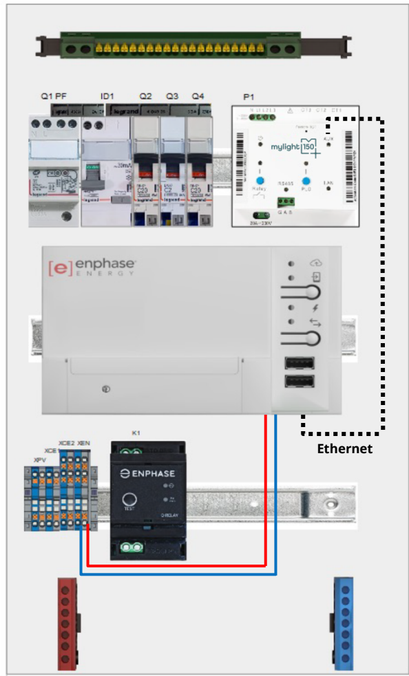
Figure 31. Schéma de principe de montage de la passerelle Envoy
