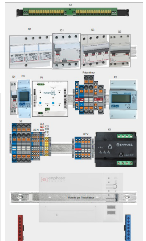
Figure 8. Cas d'utilisation typique et mise en armoire UCG-E9301-31-FR
