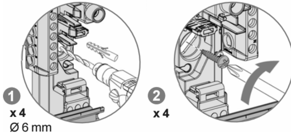
Figure 15. Montage de l'UCG sur un mur
