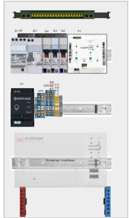
Figure 5. Cas d'utilisation typique et mise en armoire UCG-E4301-11-FR
